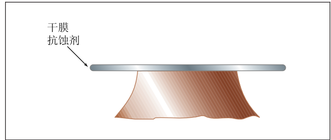
图321d 去膜前的全板电镀（干膜抗蚀剂）
