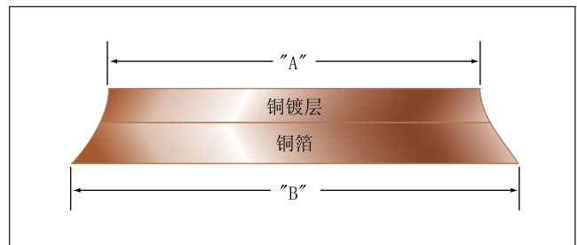
图321e 用于埋孔的内层电镀层
