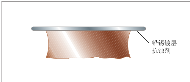
图321b 热熔前的图形电镀（干膜抗蚀剂）
