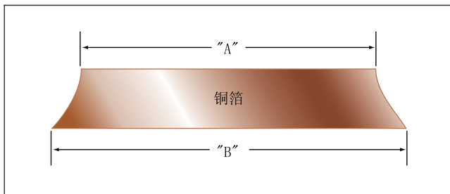
图321c 蚀刻后的内层
