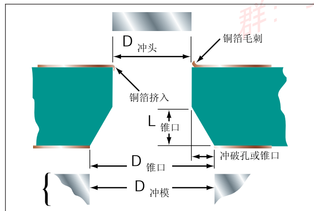
图35a 冲孔
