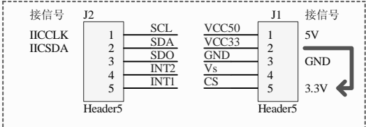
接线样例 example
